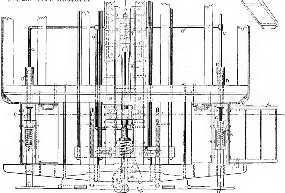
Fig. 2352. Plan.
